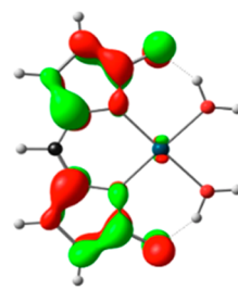
LUMO, a_2
