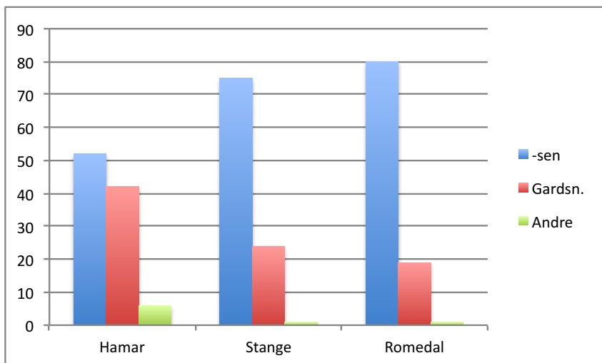
Figur 3 Hovudtypar av etternamn i dei tre kommunane – mannsnamn
