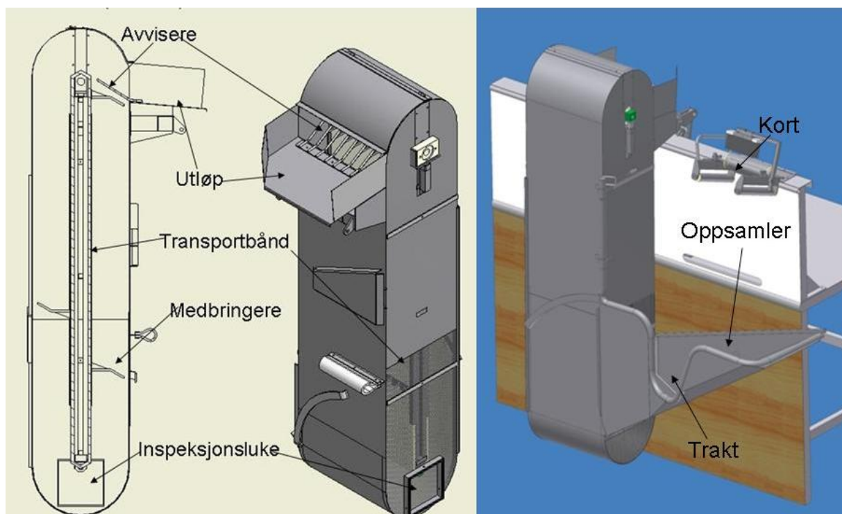
Figur 20 Skjematiske tegning av heisen på ALH med forklaringer. Levert av Borkenes Mek Verksted AS, 9475 BORKENES.
