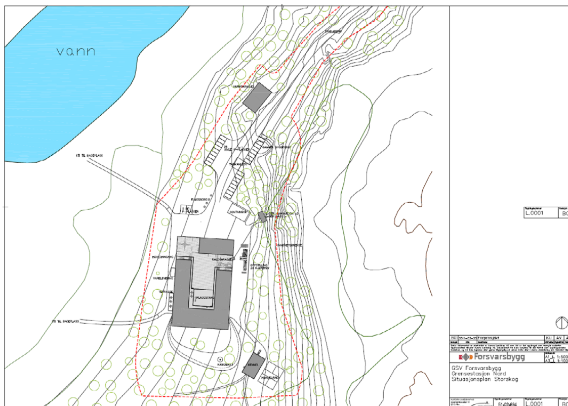
Figur 1. Situasjonsplan fra forprosjekt datert 26.03.11.
